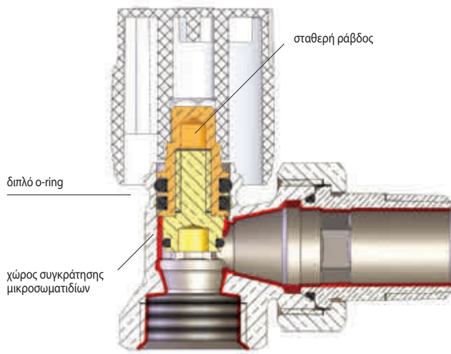
διακόπτης ανοιχτός
