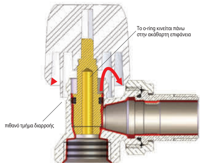
διακόπτης κλειστός
