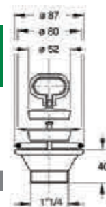
ΓΙΑ ΝΕΡΟΧΥΤΕΣ ΣΥΝΘΕΤΙΚΟΥΣ ΠΥΡΙΜΑΧΟΥΣ 1959MG54B0
