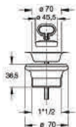
ΒΑΛΒΙΔΑ ΝΕΡΟΧΥΤΟΥ ΓΙΑ ΝΕΡΟΧΥΤΕΣ ΙΝΟΧ 1910MG64B0
