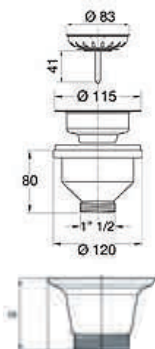
ΒΑΛΒΙΔΑ ΝΕΡΟΧΥΤΟΥ ΜΕ ΕΚΡΟΗ 3"1/2 (Ø90) 1971LX64B0
